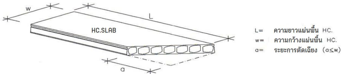
รูปที่ 22 แสดงการข้อกำหนดการตัดบากแผ่นเฉียง
